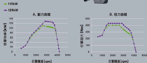
A. 高轉速時渦輪維持高峰值，馬力輸出穩定而強勁。
